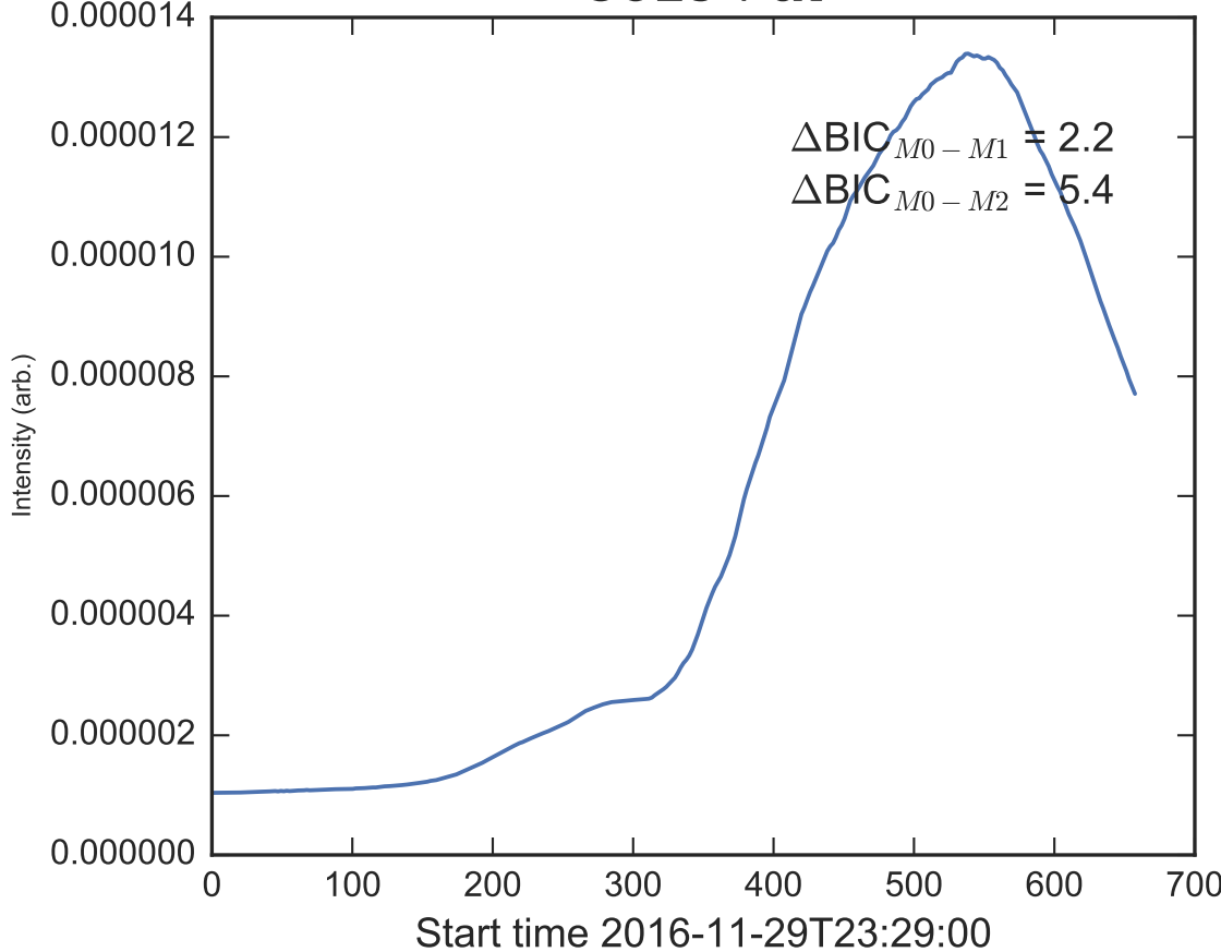
GOES 1-8Å
