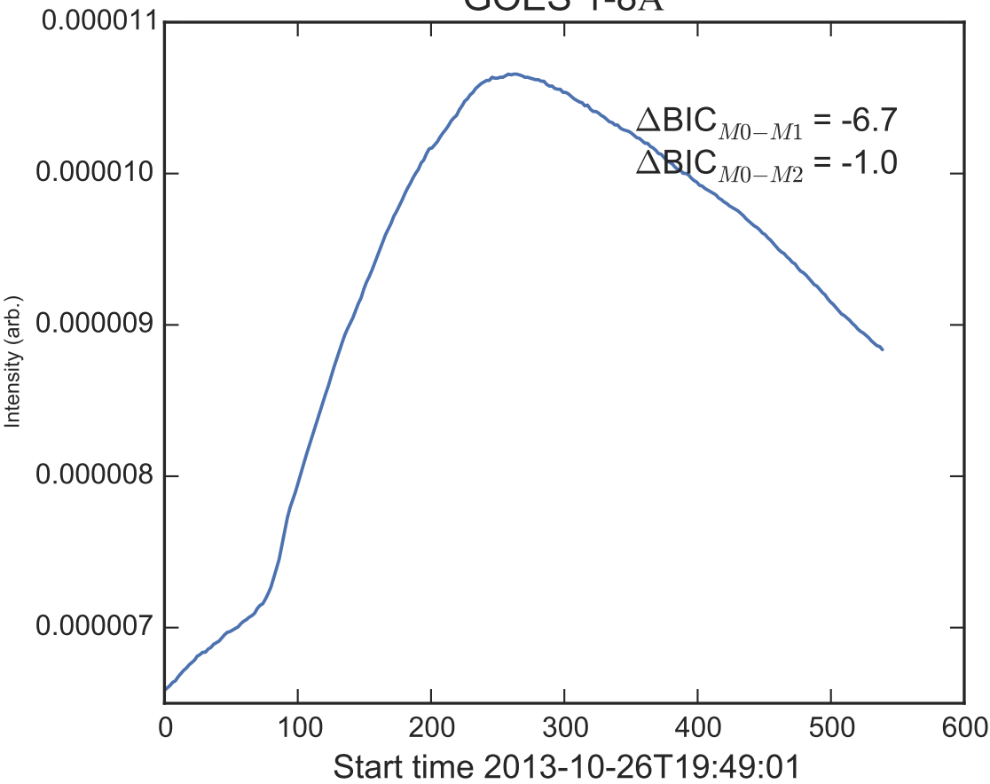
GOES 1-8Å
